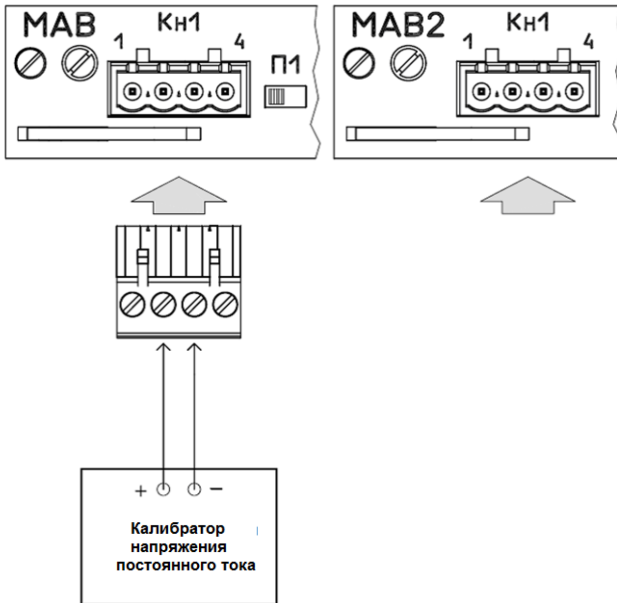
Рисунок Б.1 - Структурная схема экспериментальных исследований каналов преобразования напряжения от термоэлектрических преобразователей, унифицированных сигналов напряжения постоянного тока с диапазоном (0 – 10) mV, (0 – 20) mV, (0 – 50) mV, (0 – 100) mV и (0 – 1) V
