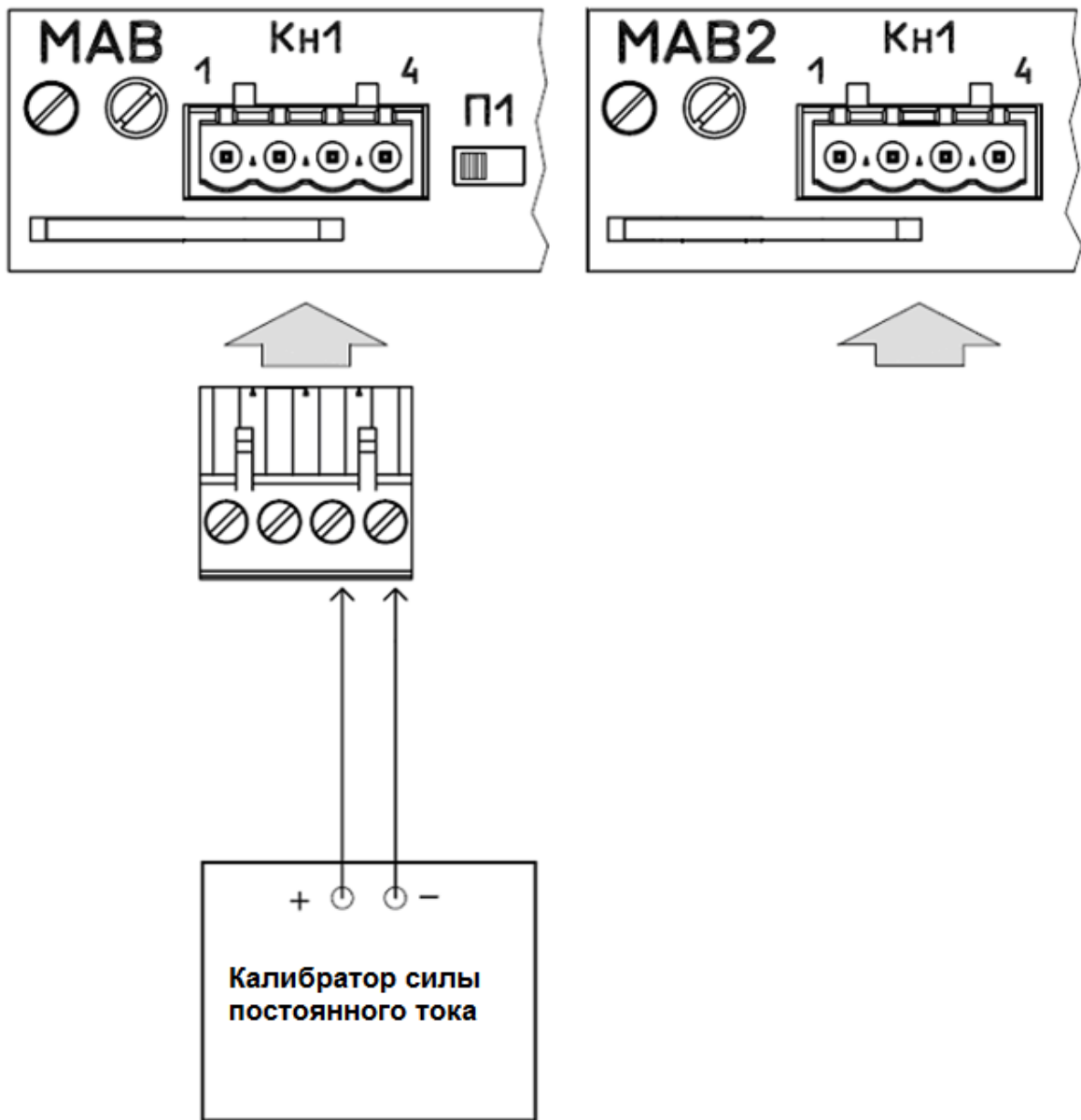
Рисунок Б. 5 - Структурная схема экспериментальных исследований каналов преобразования унифицированных сигналов силы постоянного тока с диапазоном (0 – 5) мА, (0 – 20) мА и (4 – 20) мА
