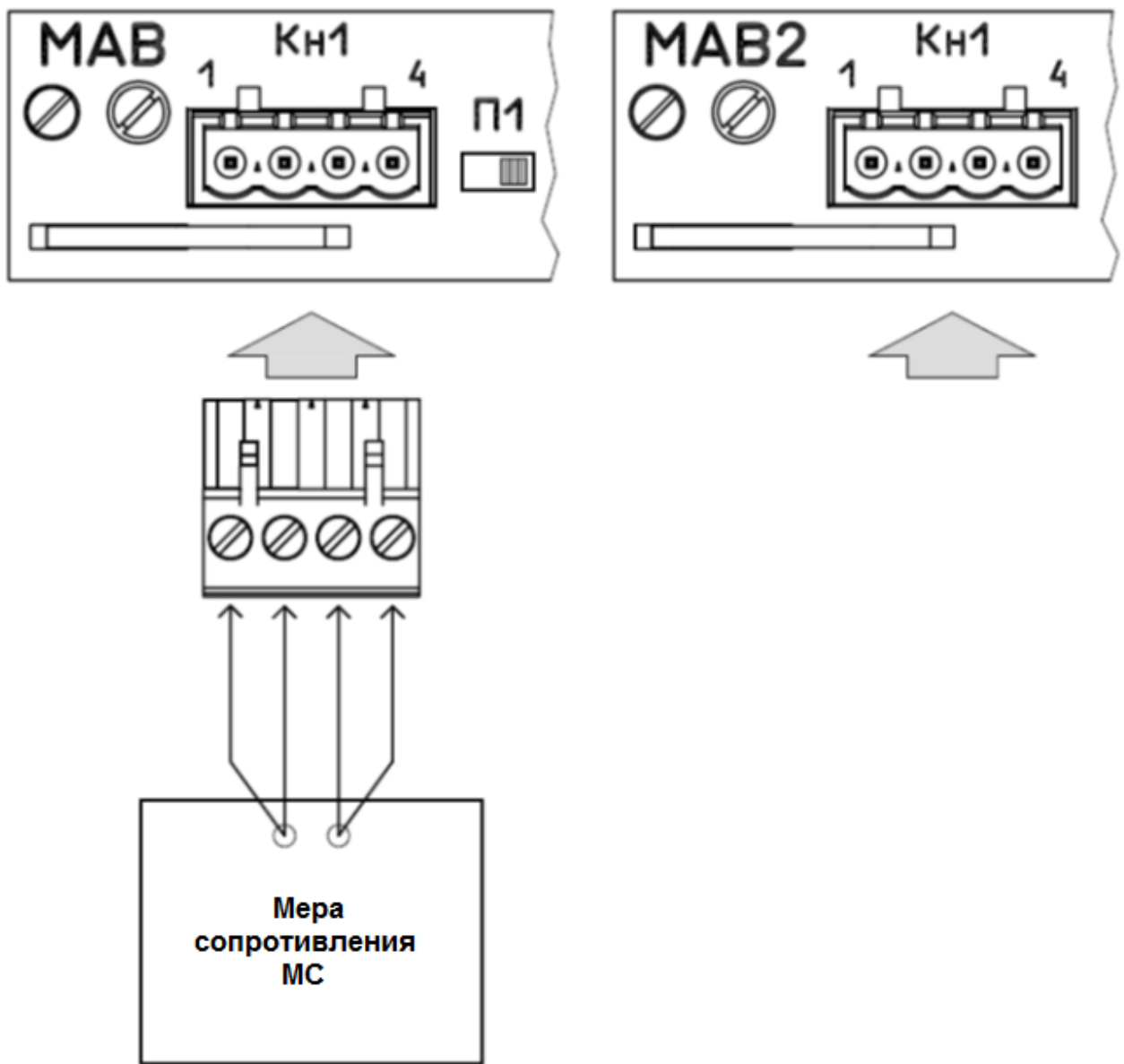
Рисунок Б. 3 - Структурная схема экспериментальных исследований каналов преобразования сопротивления для четырехпроводной схемы подключения
