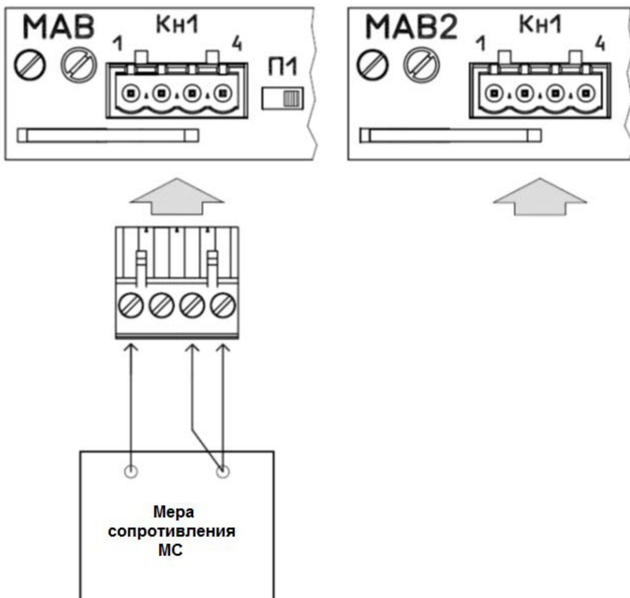
Рисунок Б. 4 - Структурная схема экспериментальных исследований каналов преобразования сопротивления для трехпроводной схемы подключения
